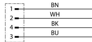
Devre şeması
