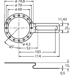
RME-11
