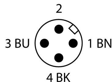
schemat obwodu
