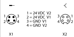
Spanningsvoeding 7/8"
