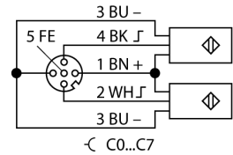
Spanningsvoeding 7/8"
