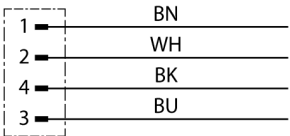
schakelplan
