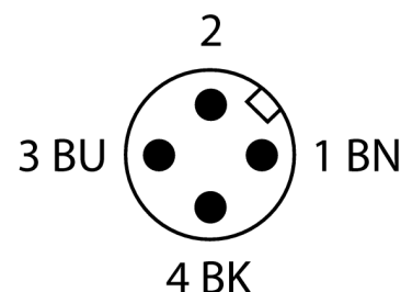
schakelplan
