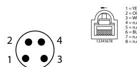
schéma de connexions
