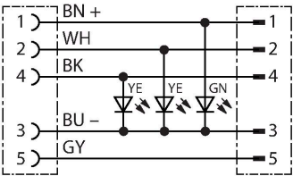
diagrama de conexiones
