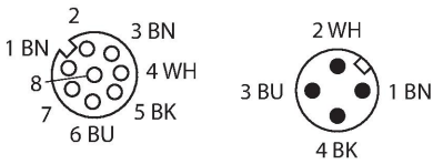
diagrama de conexiones
