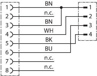
diagrama de conexiones
