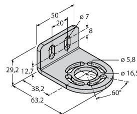
EZA-MBK-20 3072587
