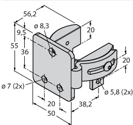
EZA-MBK-12 3071756
