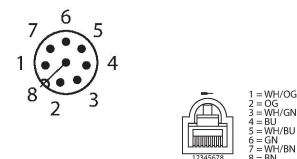
diagrama de conexiones
