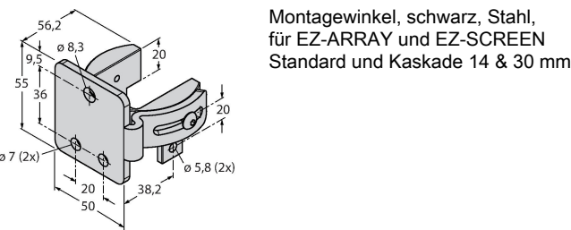
EZA-MBK-12 3071756
