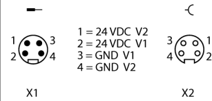
Napájecí konektor 7/8"
