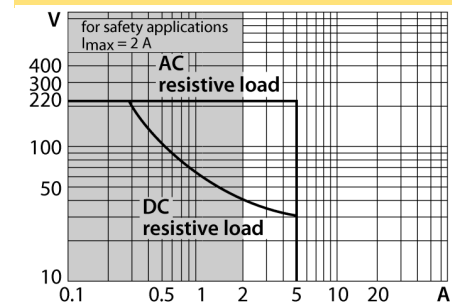
继电器输出-电流负载阈值曲线
