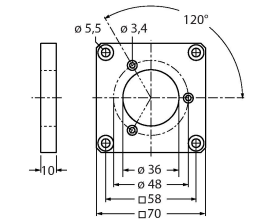
RFA-12 1544641 70 mm ( 10 mm厚 ) 方型铝制, 夹紧法兰, 轴型编码器
